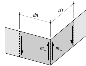
Eckkraft
