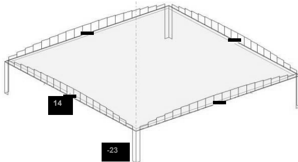
Stützkraft am Rand [kN pro Abschnitt]
