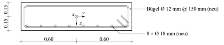
Versuchskörper N – Querschnittsgeometrie
