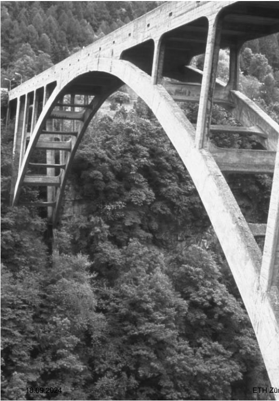
Pont de Gueuroz, Vernayaz (1934, l = 99\text{m} , L = 168\text{ m} ); Pont de Meryen, Stalden (1930, L = 118\text{ m} ). Alexandre Sarrasin.
