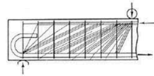
Mörsch, «Der Eisenbetonbau» (1922)
