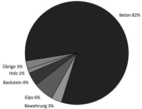
Massenbilanz Typisches Gebäude (Zürich, 2018)
