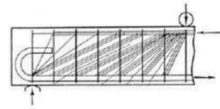
Morsch, «Der Eisenbetonbau» (1922)
