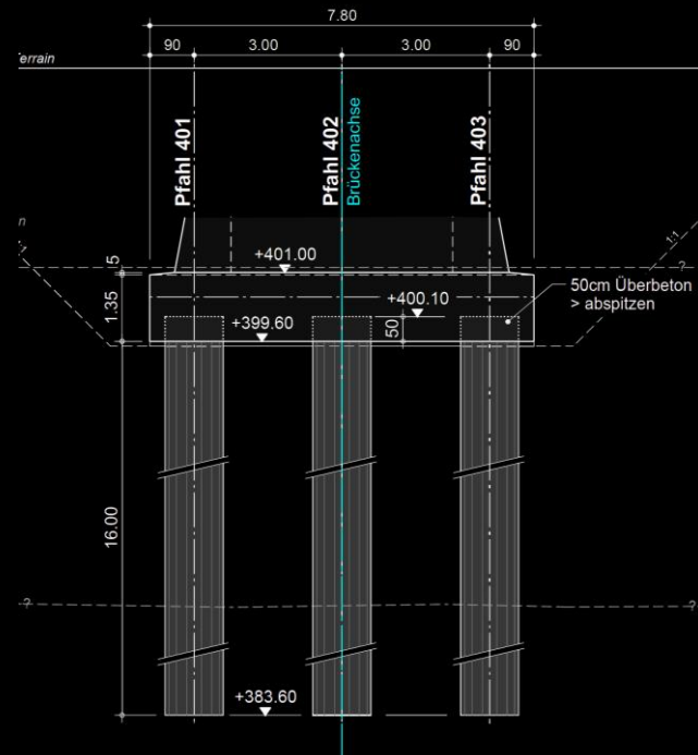
Pile cap
