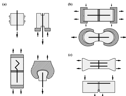
· Faserausziehversuche – schematische Versuchsanordnungen nach Bartos [16] und Gray [39]: (a) Einzelfasern mit einseitigem Verbund; (b) Einzelfasern mit beidseitigem Verbund; (c) Fasergruppen mit beidseitigem Verbund.
