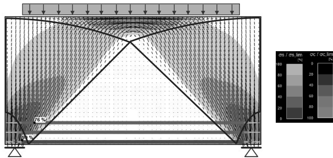
Top load: fan mechanism
